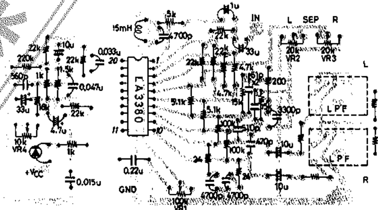
プリントパターン例 (銅箔面) 130×65 mm 2
